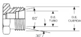
MACHO DIN CÓNICO 24° 6711
