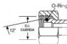
HEMBRA DIN CÓNICO 24° CON O-RING (FDLORX/FDHORX)
