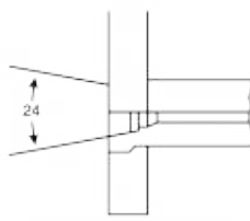
BRIDA HEMBRA
