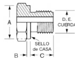
MACHO TIPO B
