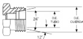
MACHO DIN CÓNICO 24° 2353 (MDL/MDH)
