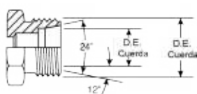
MACHO FRANCÉS 24°
