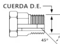
MACHO GIRATORIO SAE ABOCINADO INVERTIDO (MIX)
