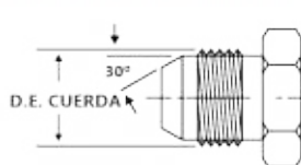
MACHO SÓLIDO (MZ)
