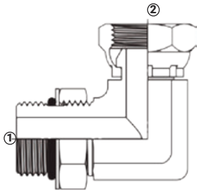
(1) Macho SAE O-ring (2) Hembra NPSM giratoria SAE 140257
