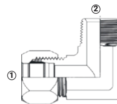
(1) Tubing Macho (2) Macho NPTF
