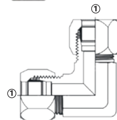
(1) Tubing (2) Tubing
