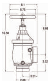
válvula de ángulo ranura x Hembra
