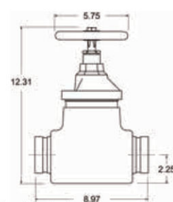
válvula de globo ranura x ranura
